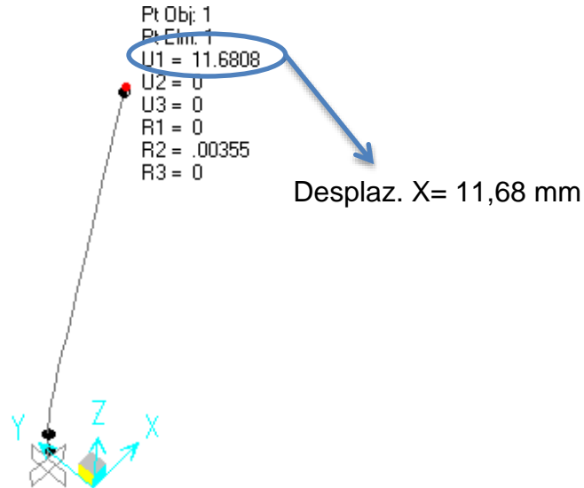
Figura 12.1.2: Desplazamiento lateral debido al viento ( W_x ), (mm).
