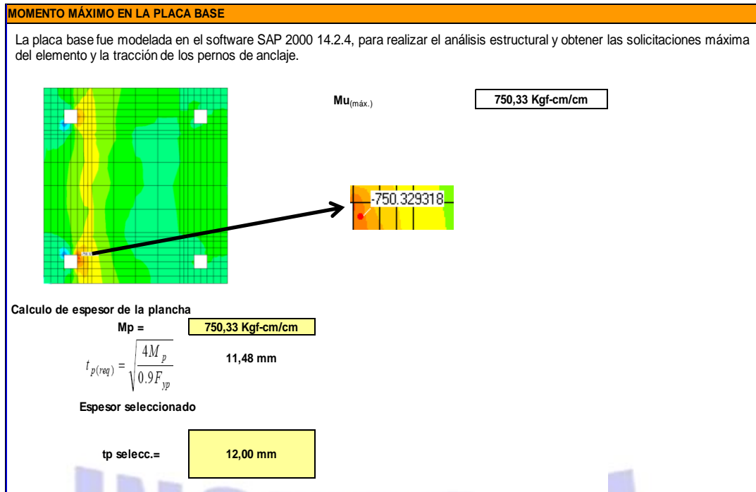
Figura 12.2.1: Hoja de cálculo – Diseño de espesor de placa base. (Fuente: Elaboración propia).
