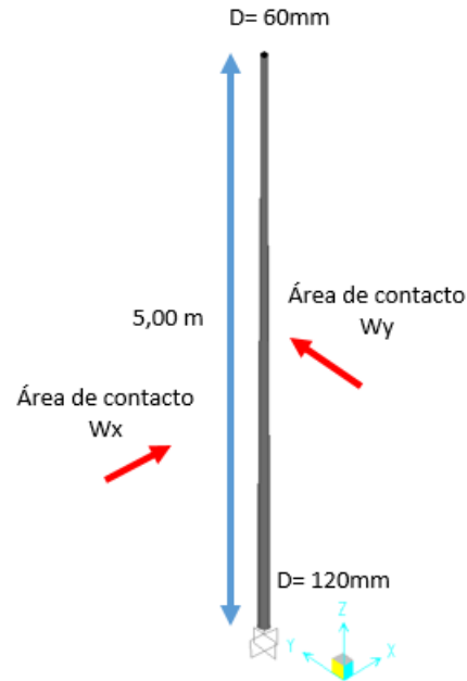
Figura 10.1: Áreas de contacto del viento a la estructura del poste (Fuente: Elaboración propia).
