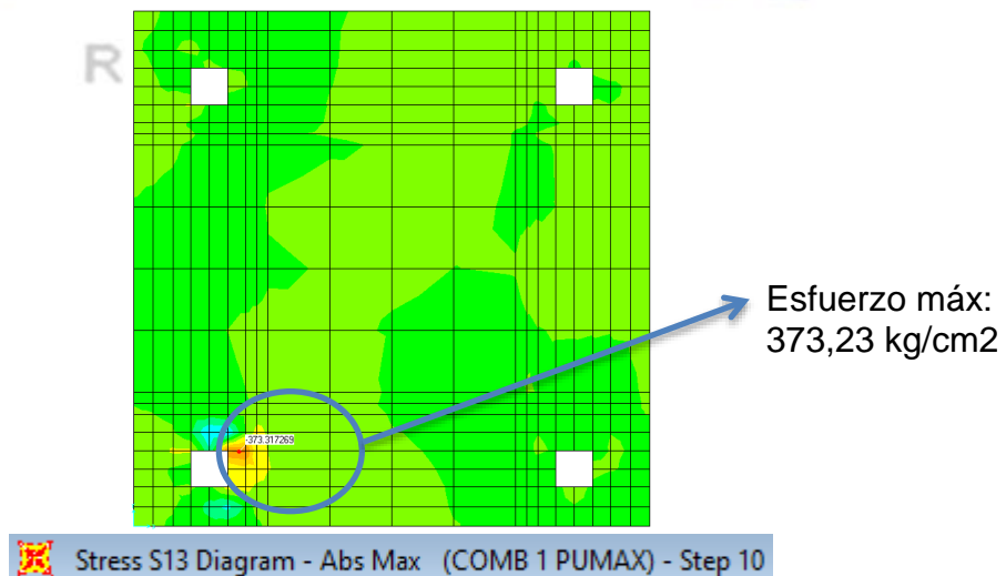
Figura 12.2.2: Esfuerzo en la placa base. (Fuente: Modelo en el programa SAP2000 V14.2.4).
